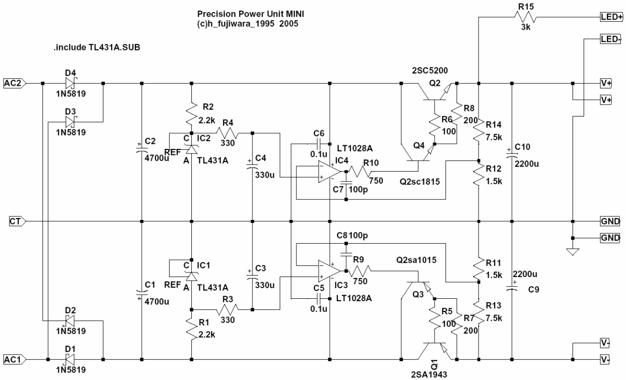
図 回路図
