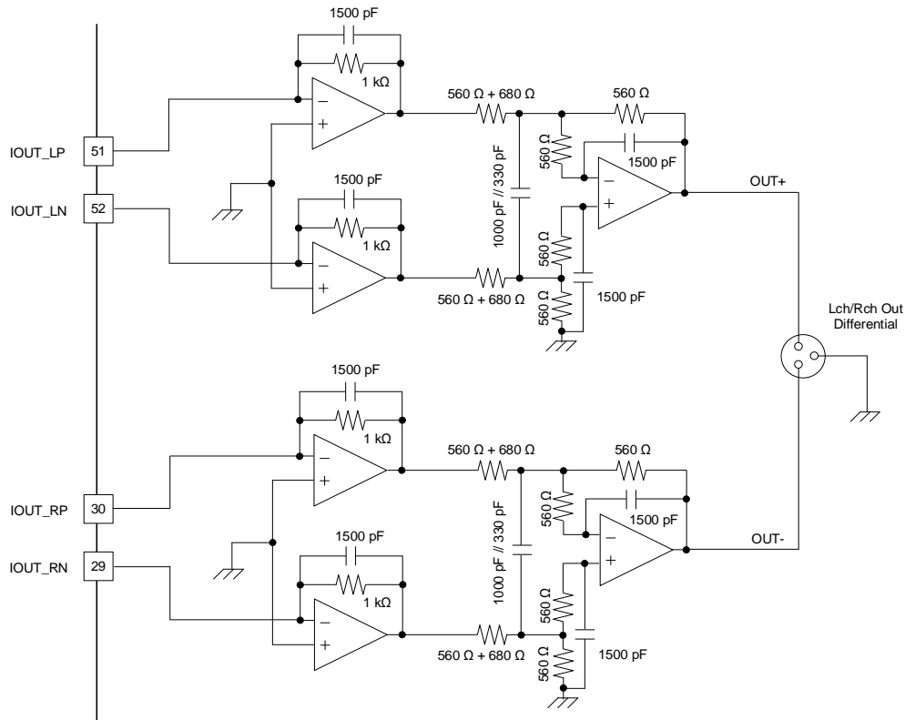
Figure 41. モノモード x2 - B 設定時の応用回路
