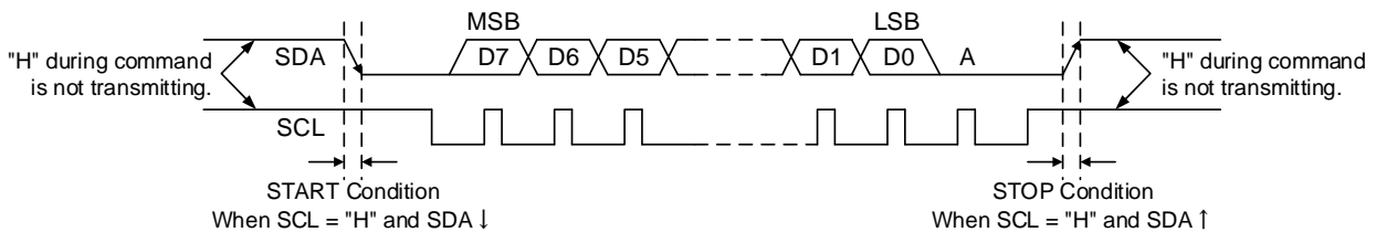
Figure 14. スタートストップ規定
