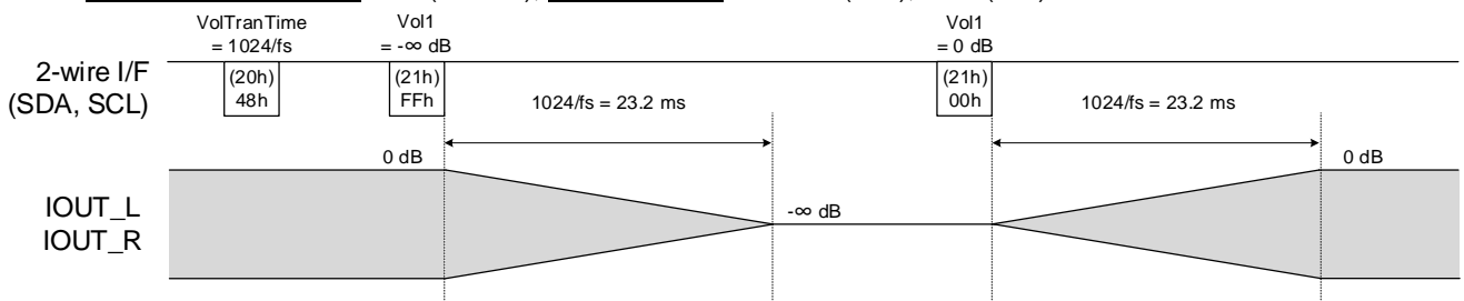
Figure 21. ボリューム切り替え例
