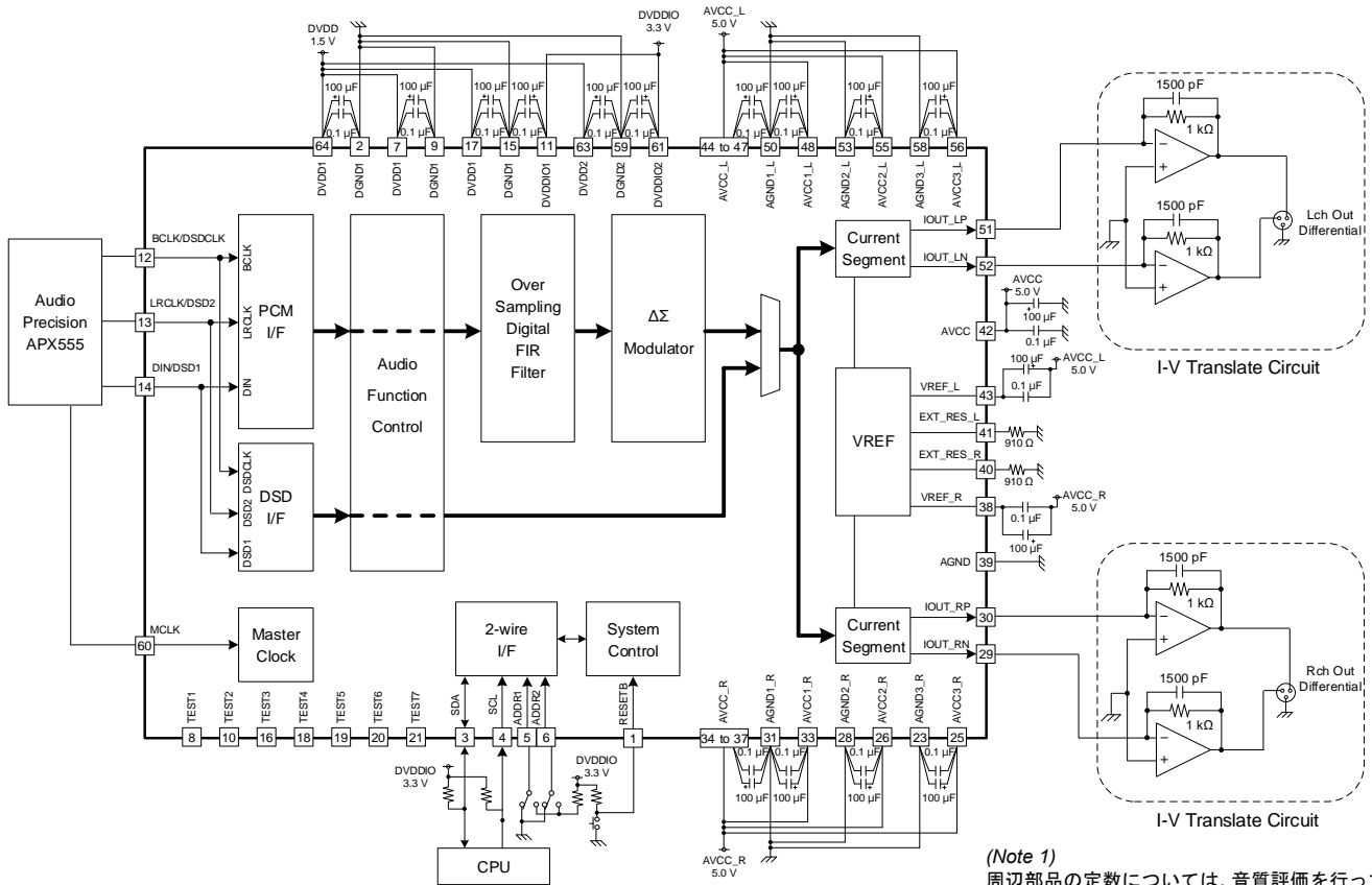
Figure 5. 測定回路図
