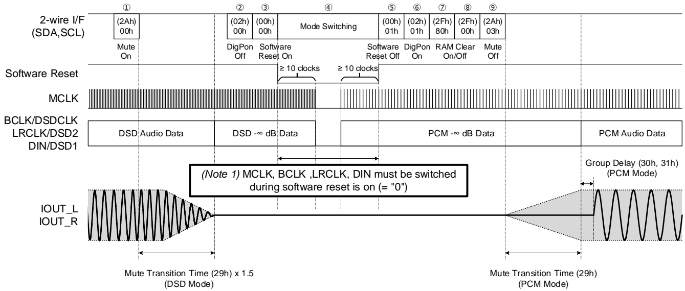
Figure 36. DSD から PCM へのモード切り替えシーケンス
