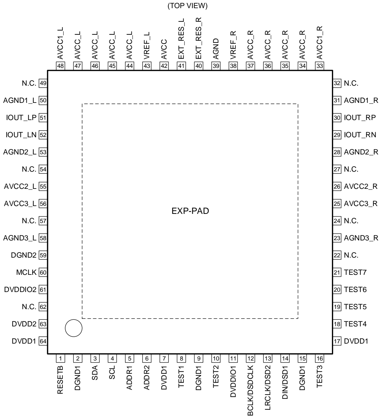
Figure 2. 端子配置図
