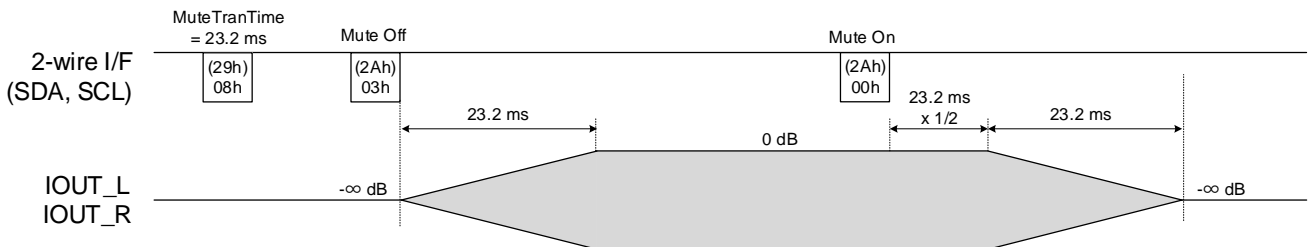
Figure 23. ミュートのオン/オフ例 (DSD モード)
