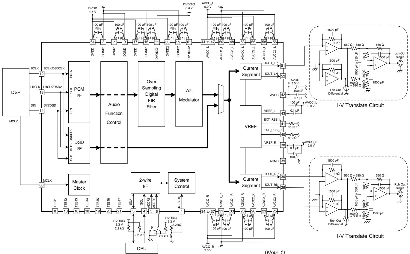
Figure 38. 応用回路図
