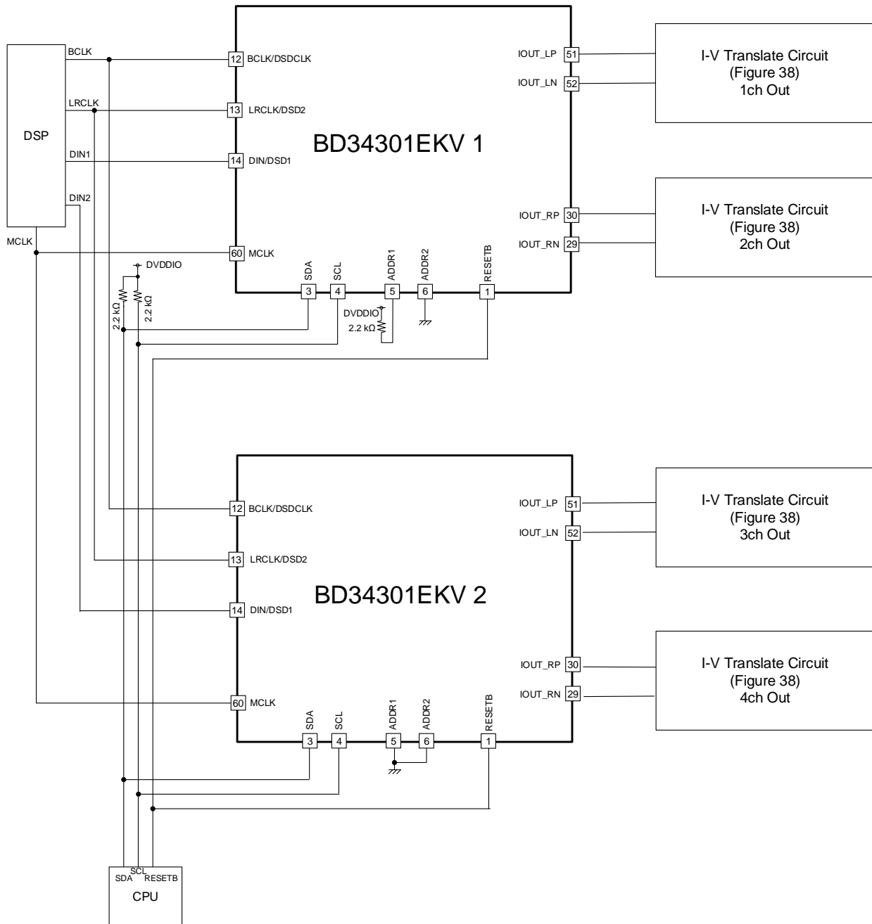
Figure 41. 4ch 出力時の応用回路
