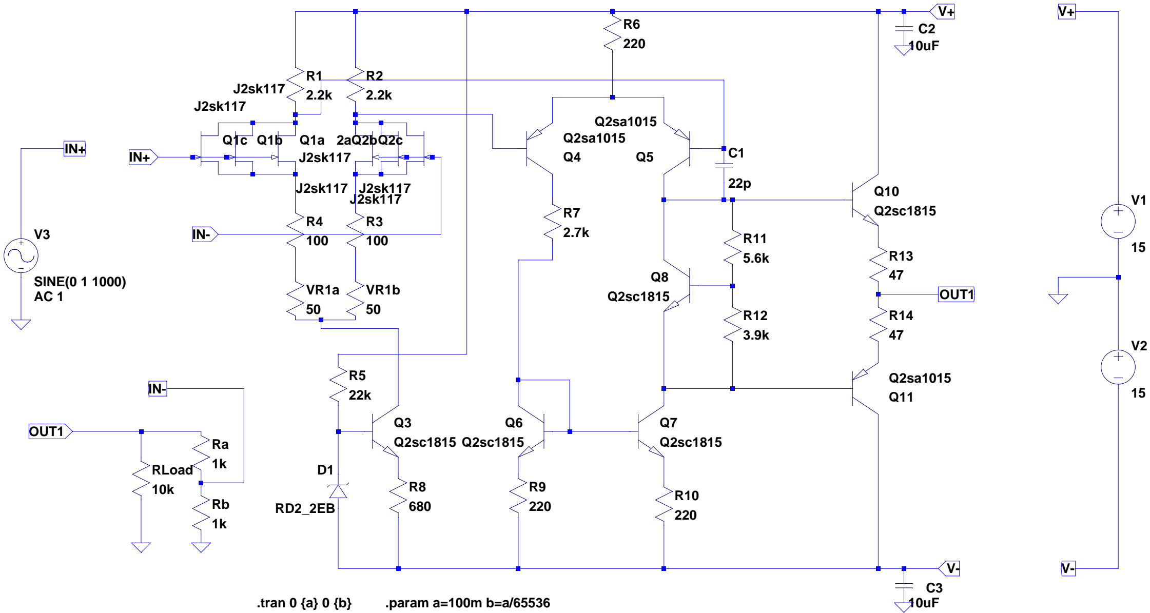
Descreate OP amplifier module A-9
