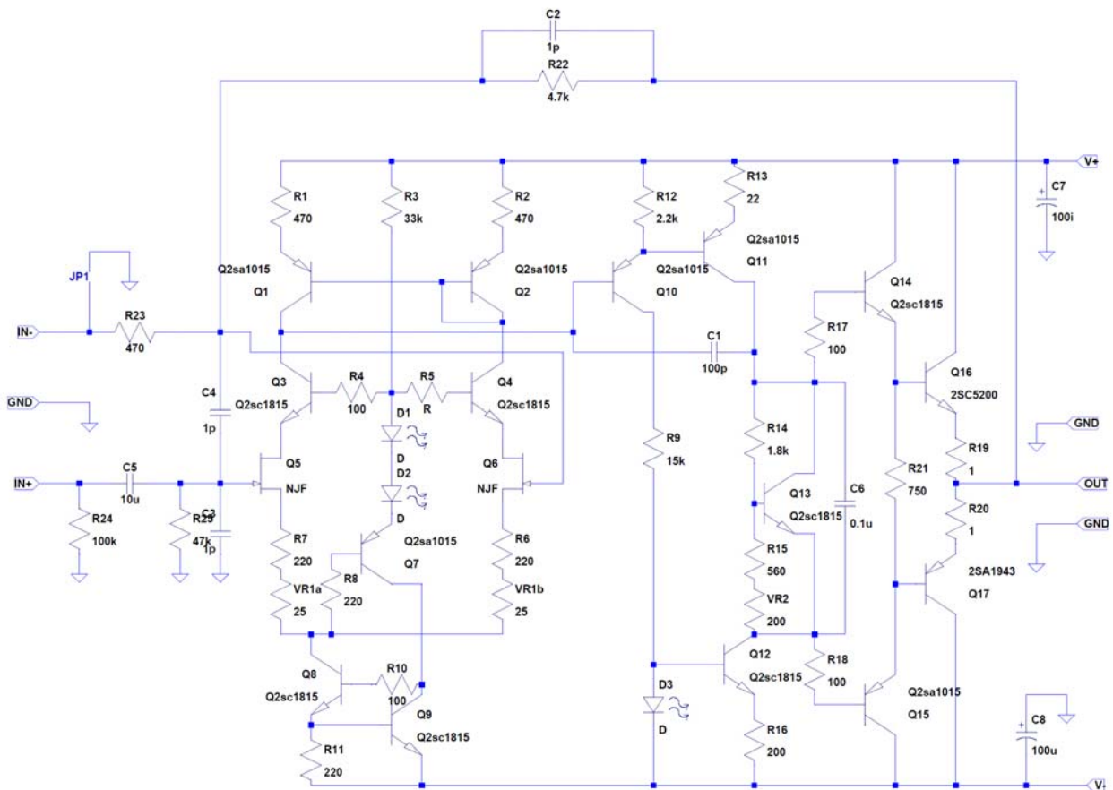
(a)全体回路
