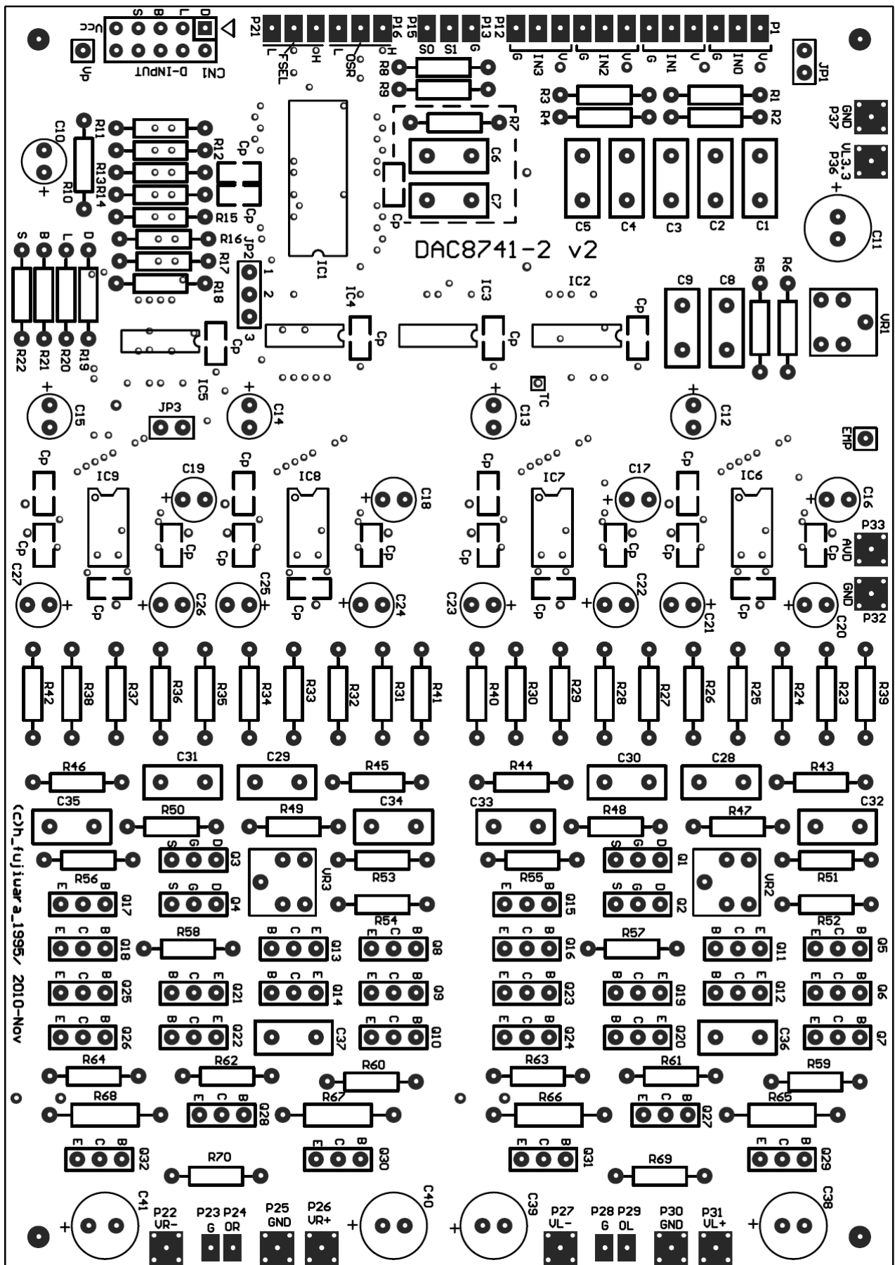
(a) シルクパターン (V2 基板)
