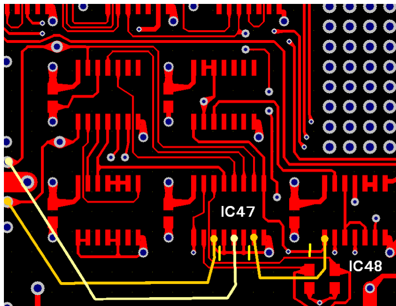
図 ジャンパーを3本接続
