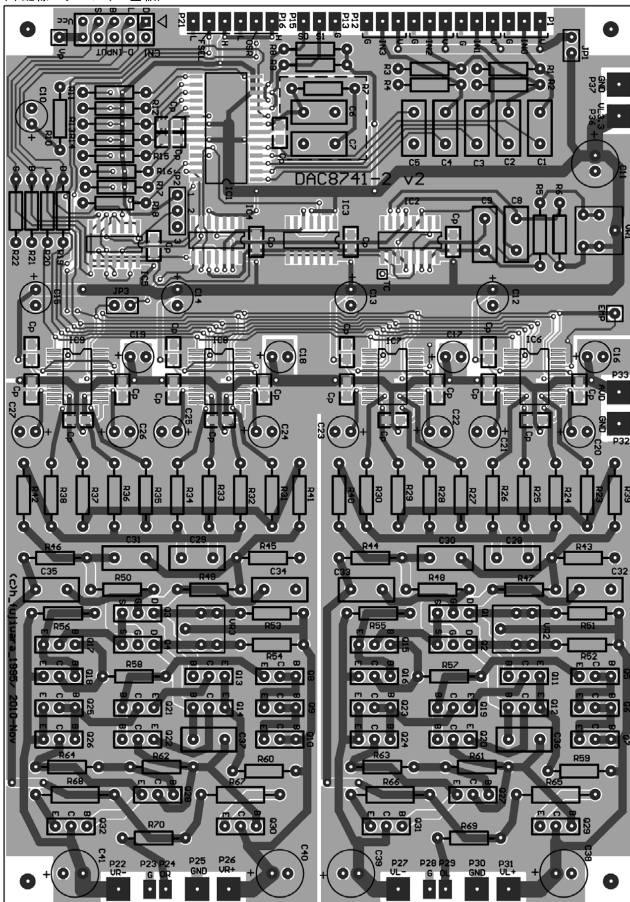
(b) 配線パターン (V2 基板)
