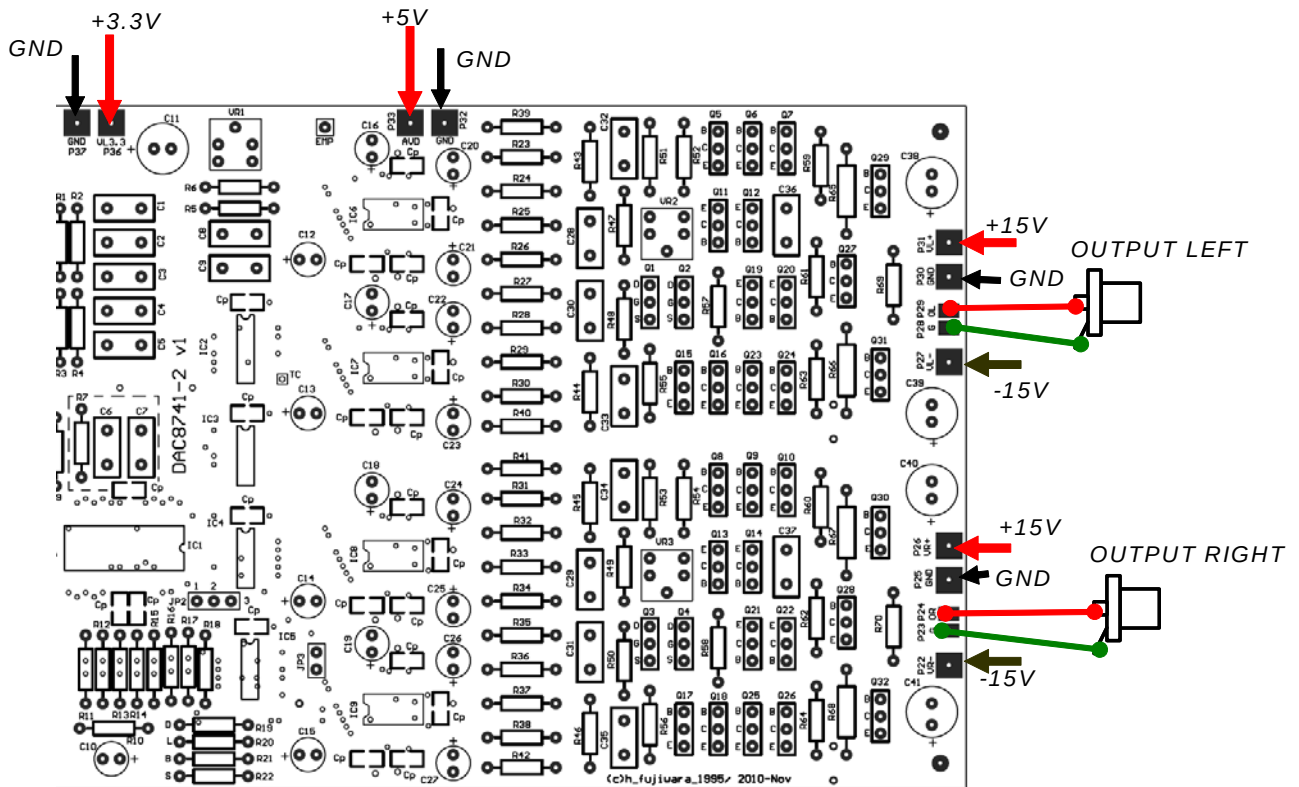
図 電源およびオーディオ出力コネクタとの接続
