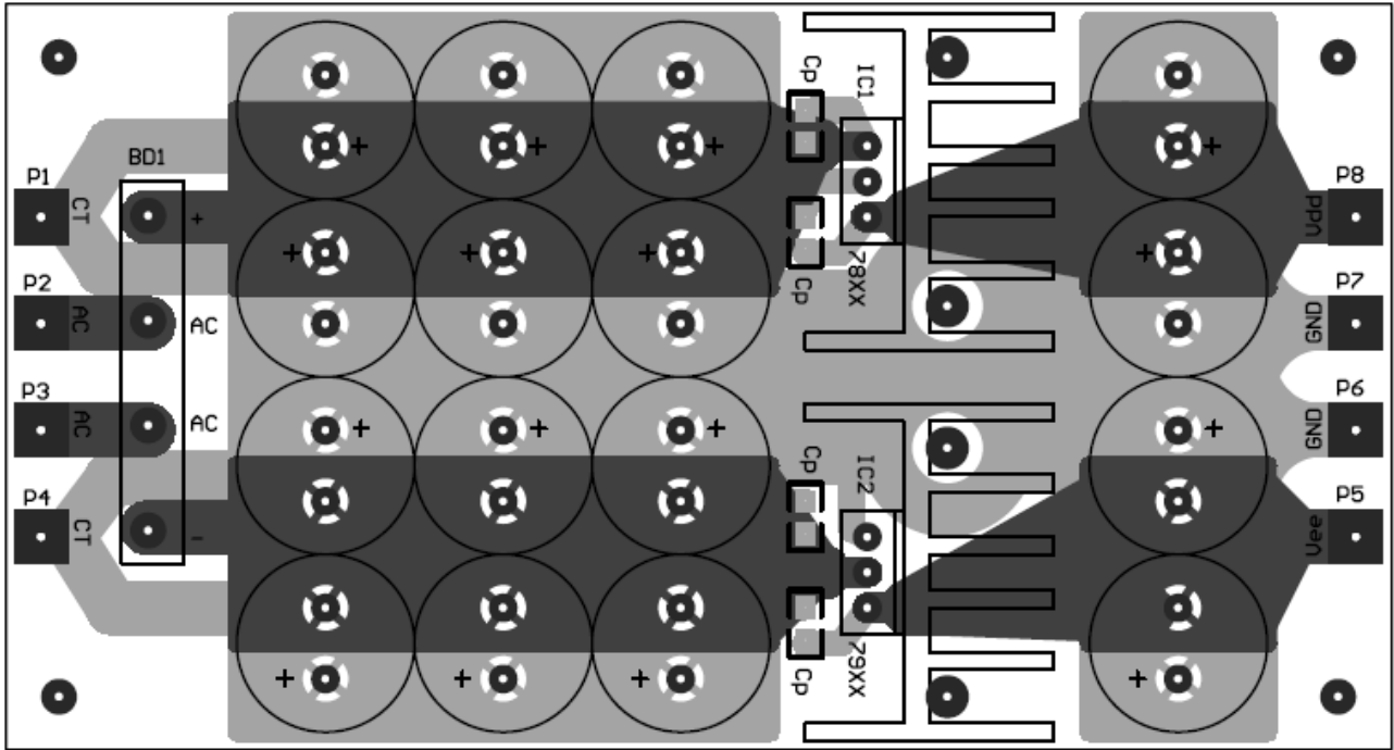
図 基板パターン
