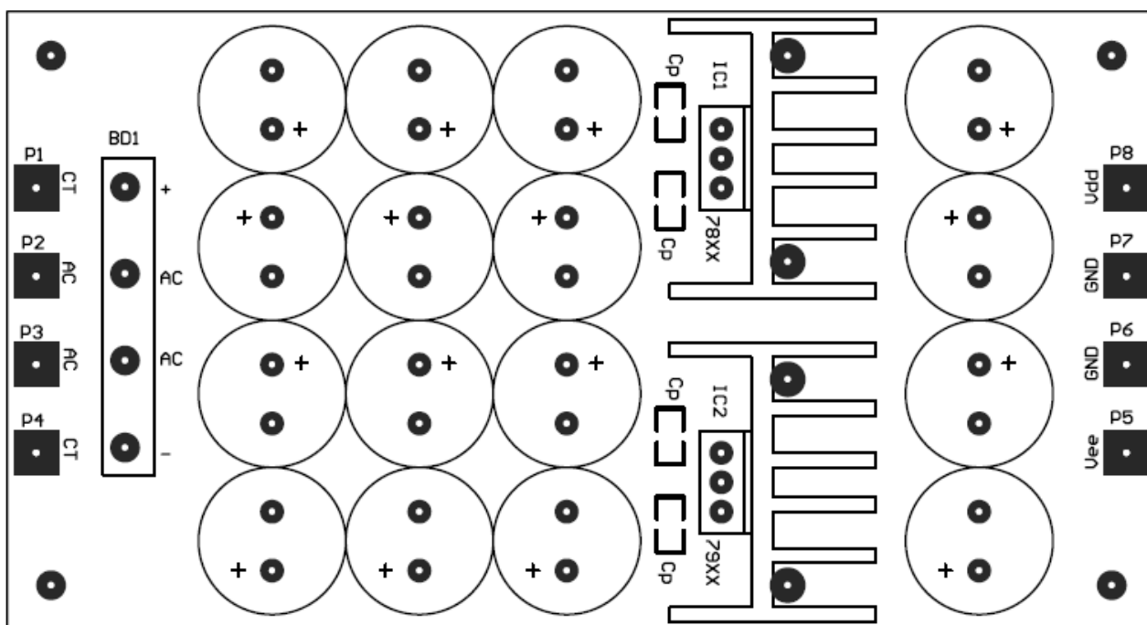
図 基板シルク (基板サイズ : 99×53mm)
